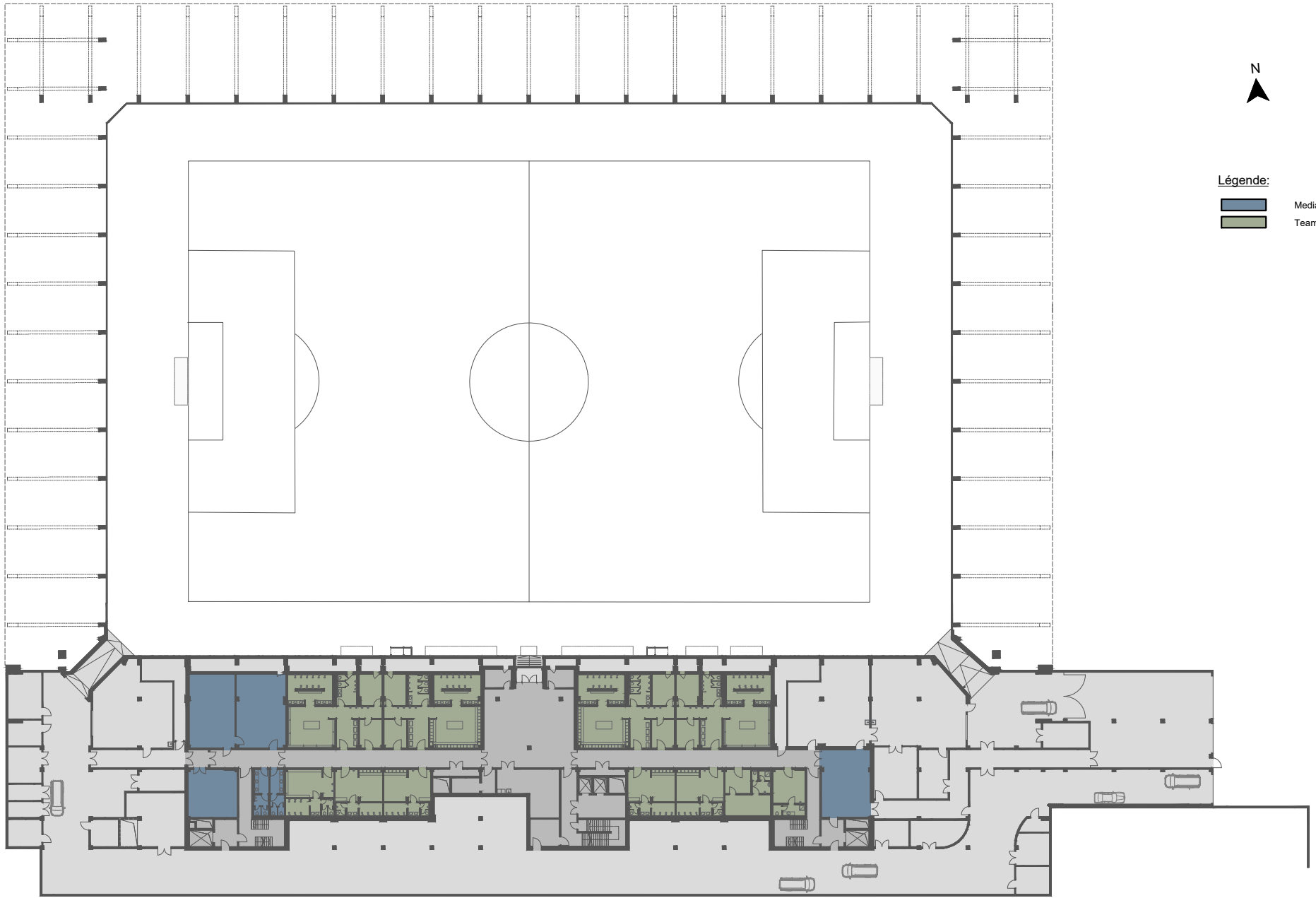
PLAN DU SOUS-SOL
